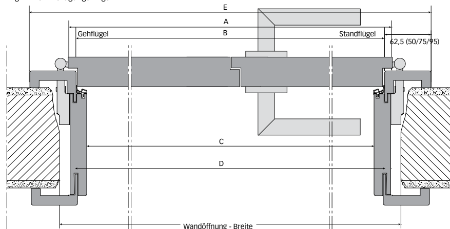
2-flg. Einzelanfertigungszarge
